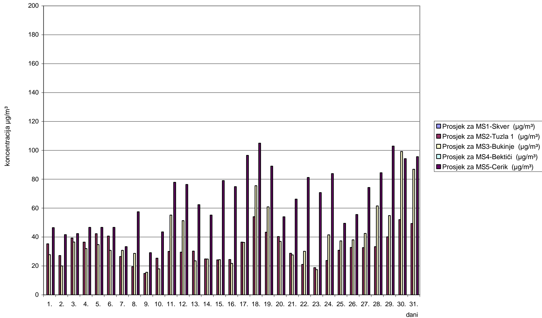
Slika 2. Grafički prikaz prosječnih dnevnih vrijednosti azotdioksida (NO 2 ) za mjesec oktobar/listopad 2011. godine
