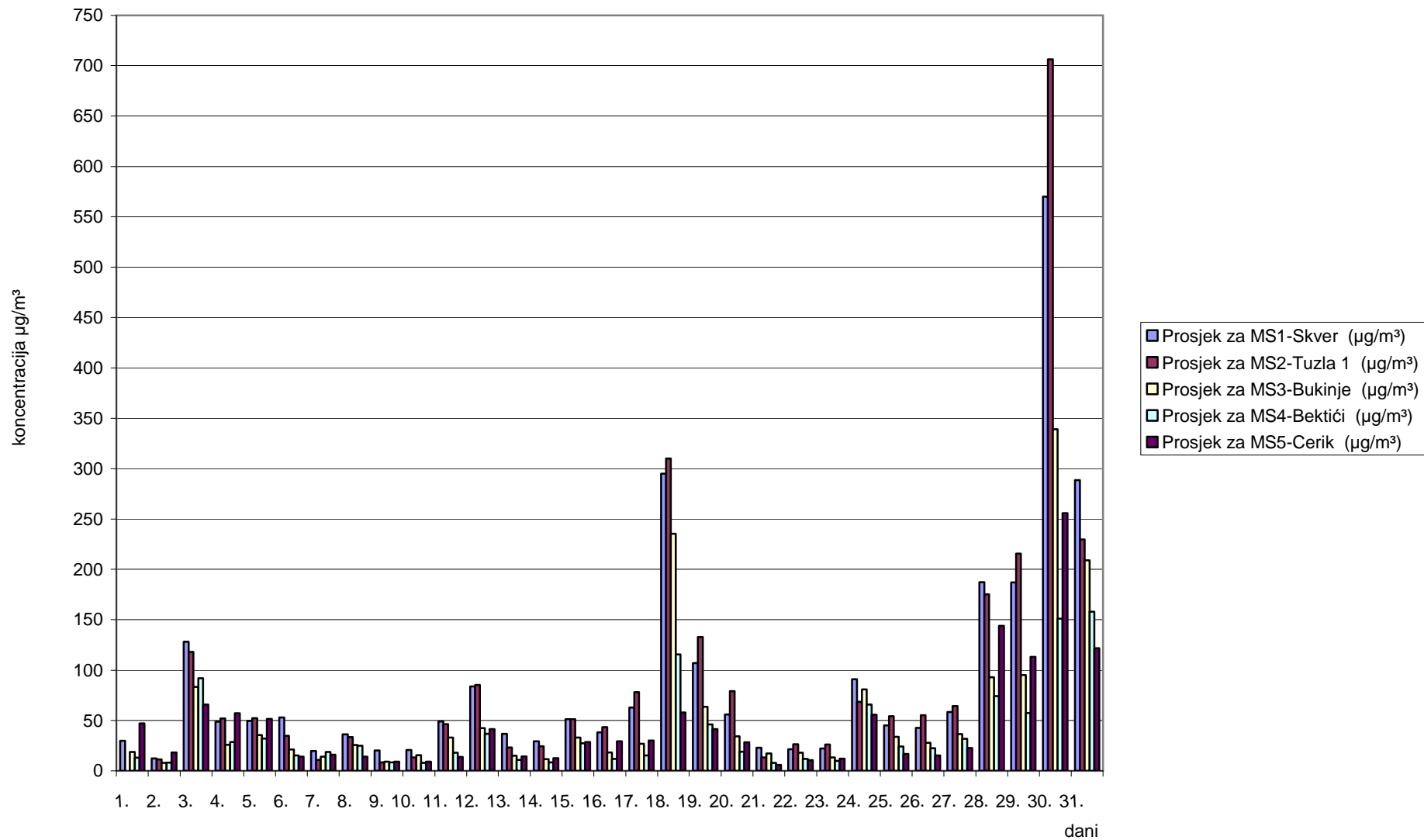
Slika 1. Grafički prikaz prosječnih dnevnih vrijednosti sumpordioksida (SO 2 ) za mjesec oktobar/listopad 2011. godine
