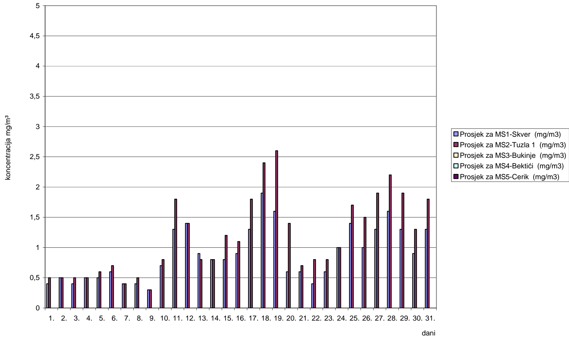
Slika 3. Grafički prikaz prosječnih dnevnih vrijednosti ugljenmonoksida (CO) za mjesec oktobar/listopad 2011. godine
