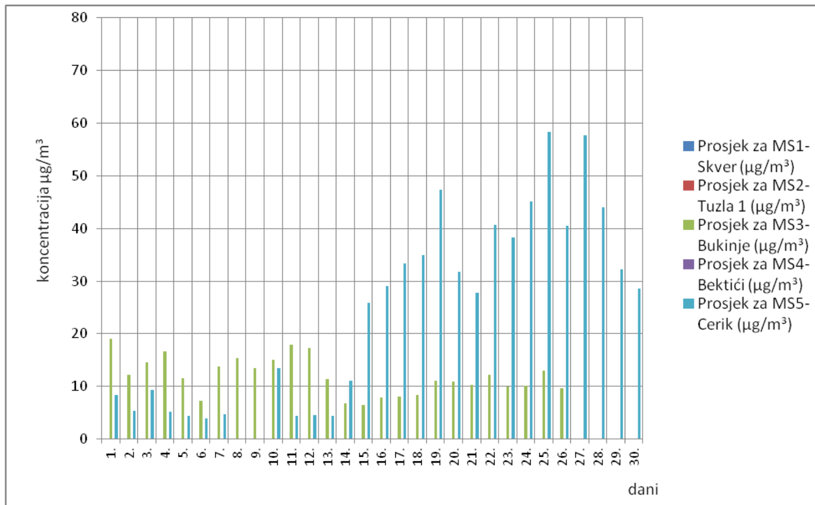
Slika 4. Grafički prikaz prosječnih dnevnih vrijednosti ozona (O 3 ) za mjesec septembar/rujan 2012. godine
