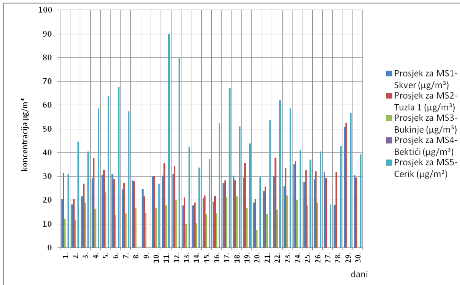
Slika 2. Grafički prikaz prosječnih dnevnih vrijednosti azotdioksida (NO 2 ) za mjesec septembar/rujan 2012. godine
