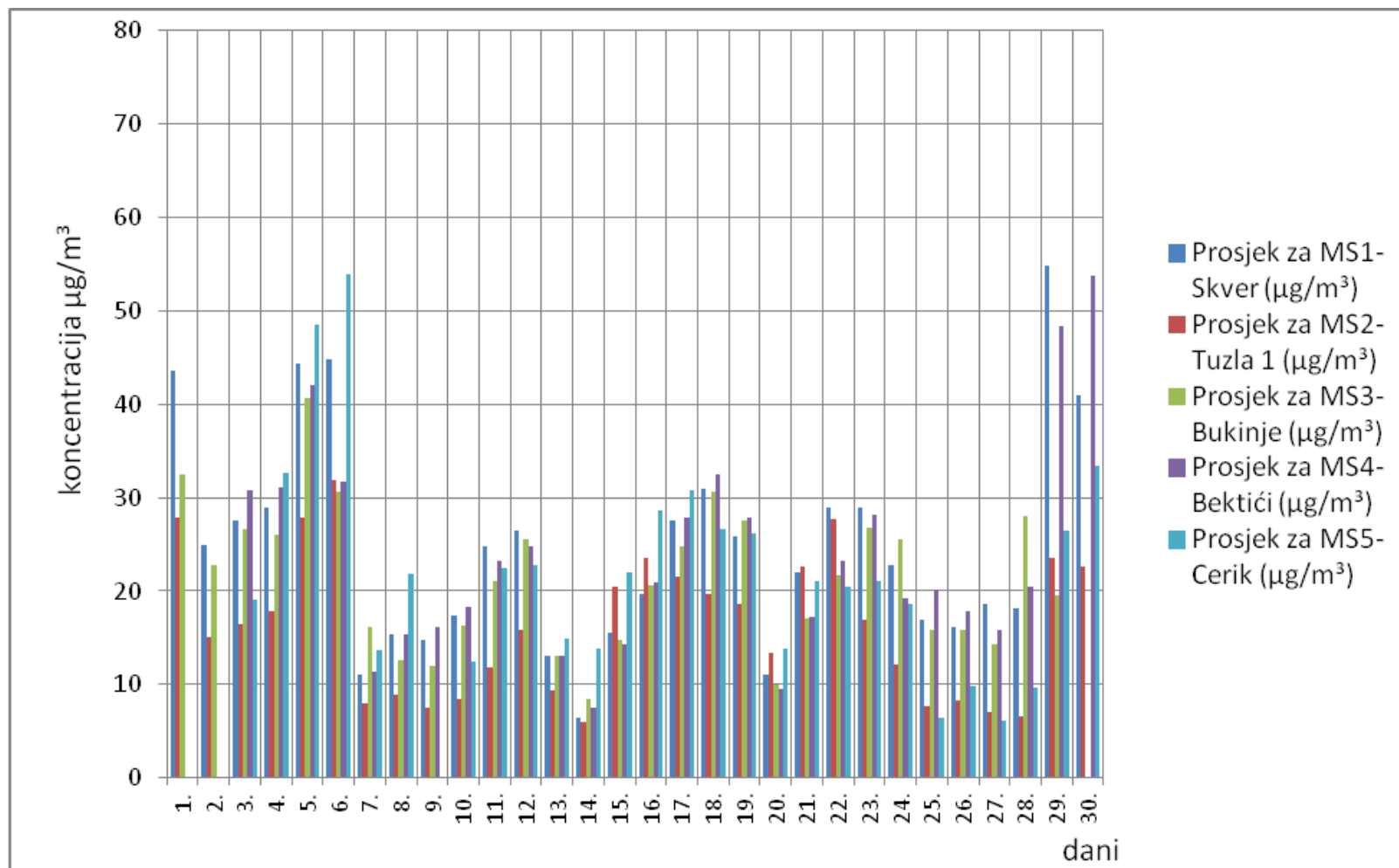
Slika 5. Grafički prikaz prosječnih dnevnih vrijednosti suspendovanih čestica (PM 2,5 ) za mjesec septembar/rujan 2012. godine
