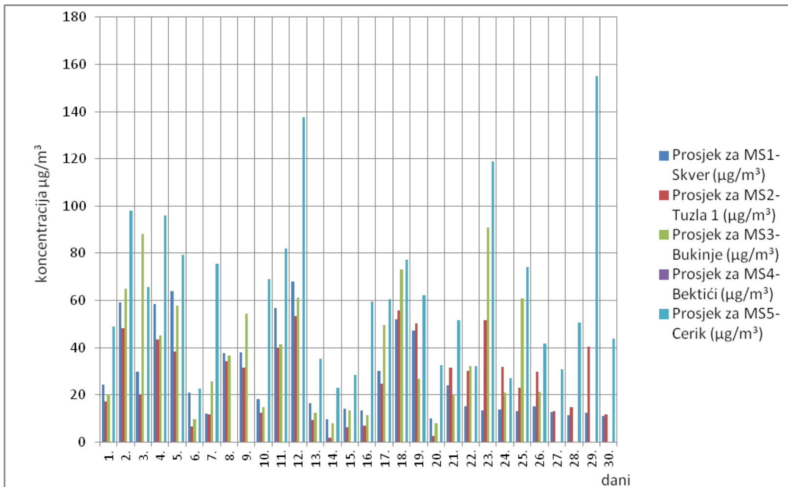
Slika 1. Grafički prikaz prosječnih dnevnih vrijednosti sumpordioksida (SO 2 ) za mjesec septembar/rujan 2012. godine
