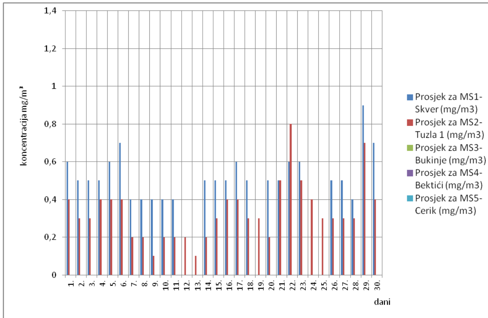
Slika 3. Grafički prikaz prosječnih dnevnih vrijednosti ugljenmonoksida (CO) za mjesec septembar/rujan 2012. godine
