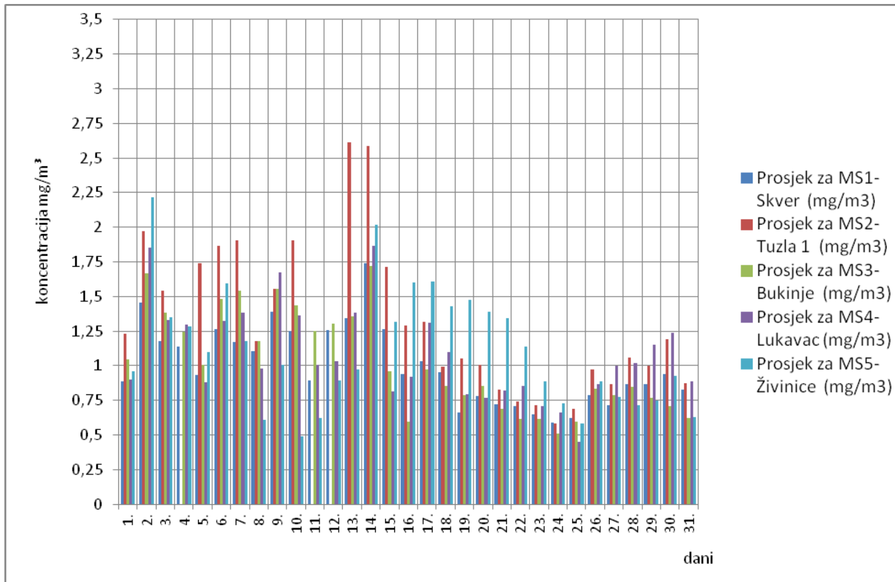
Slika 3. Grafički prikaz prosječnih dnevnih vrijednosti ugljenmonoksida (CO) za mjesec mart/ožujak 2017. godine
