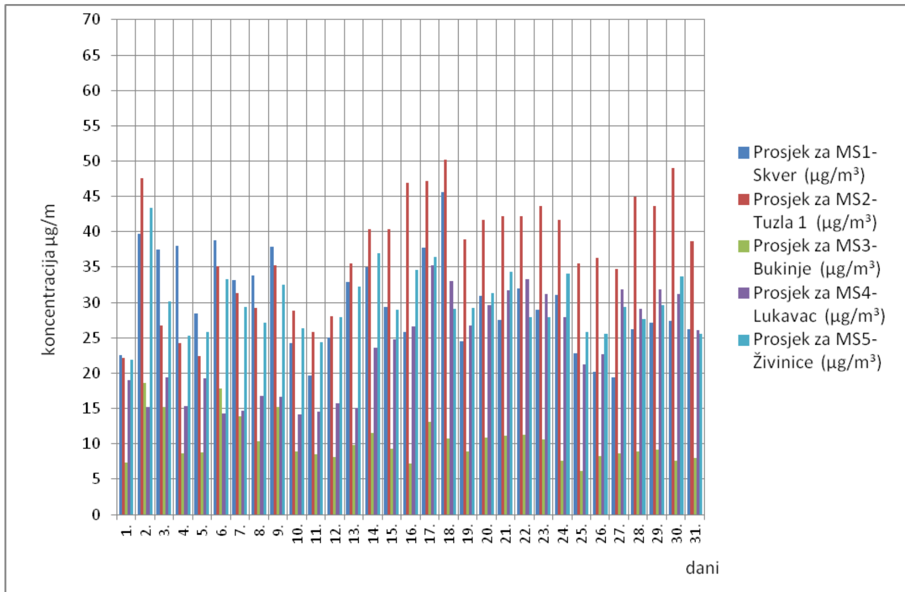
Slika 2. Grafički prikaz prosječnih dnevnih vrijednosti azotdioksida (NO 2 ) za mjesec mart/ožujak 2017. godine
