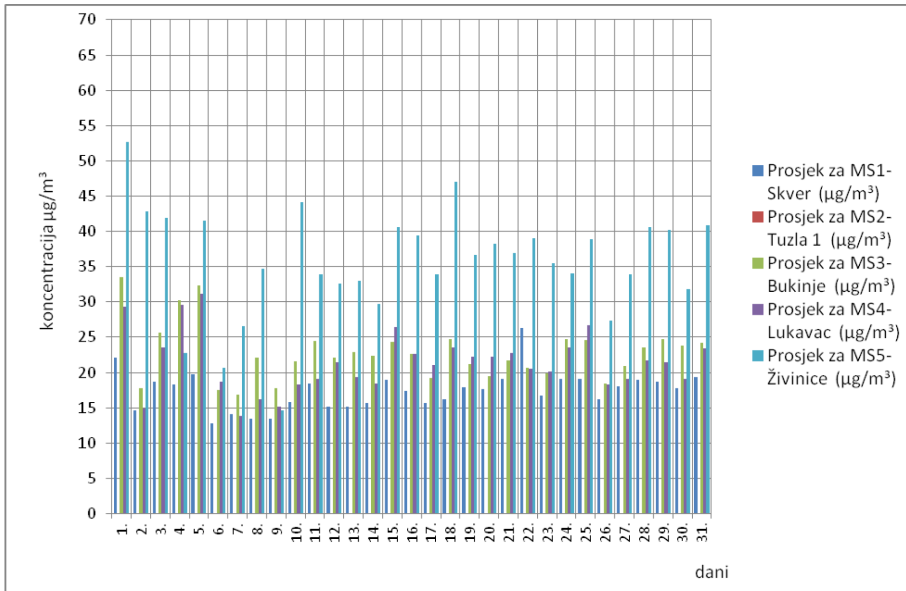
Slika 4. Grafički prikaz prosječnih dnevnih vrijednosti ozona ( \text{O}_3 ) za mjesec mart/ožujak 2017. godine
