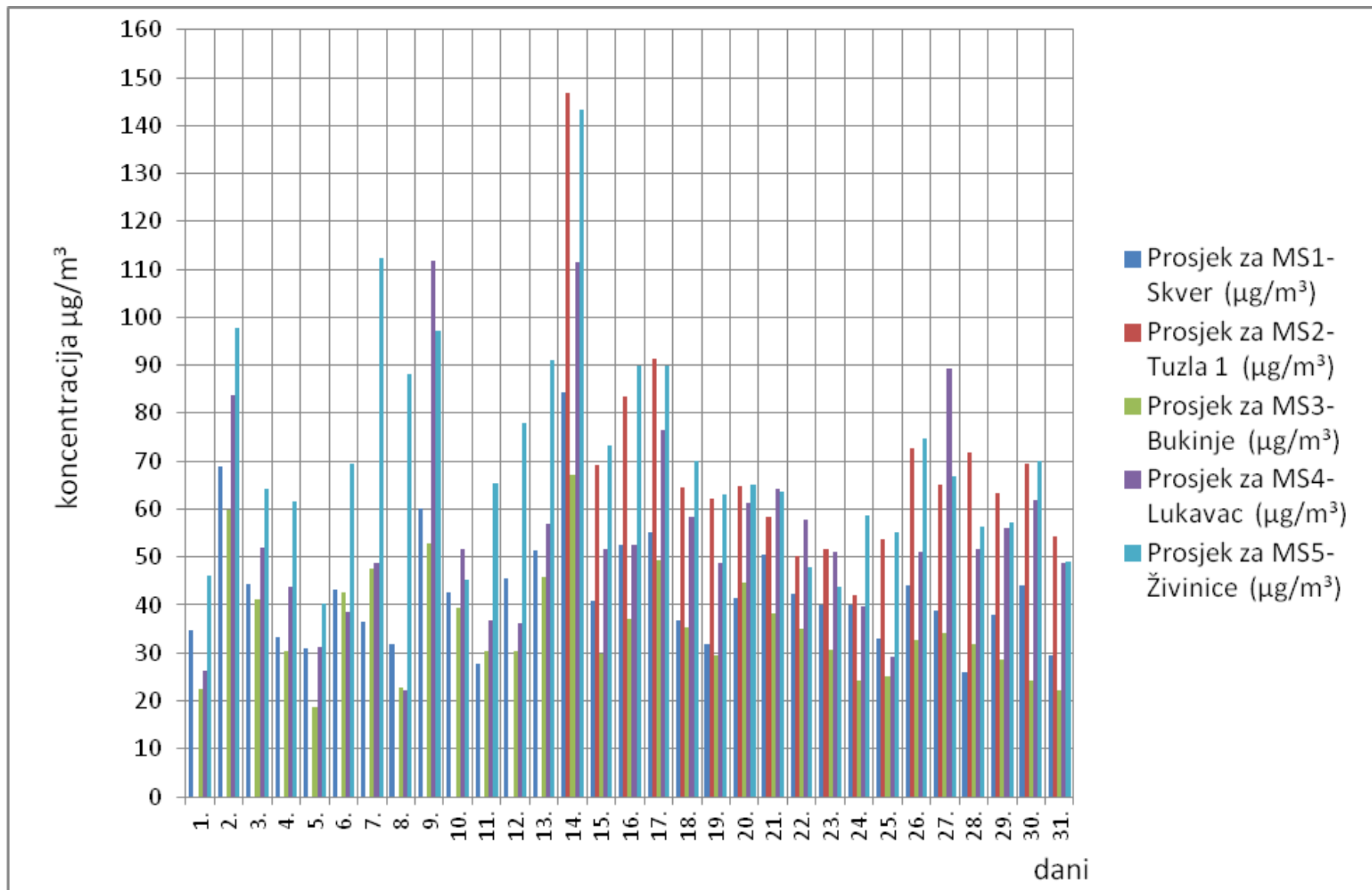
Slika 5. Grafički prikaz prosječnih dnevnih vrijednosti suspendovanih čestica (PM 2,5 ) za mjesec mart/ožujak 2017. godine
