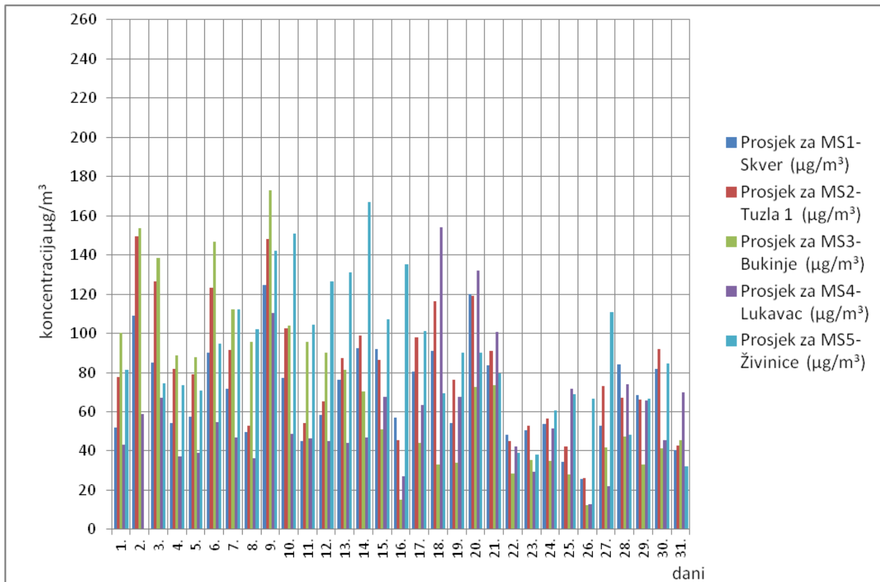
Slika 1. Grafički prikaz prosječnih dnevnih vrijednosti sumpordioksida (SO 2 ) za mjesec mart/ožujak 2017. godine
