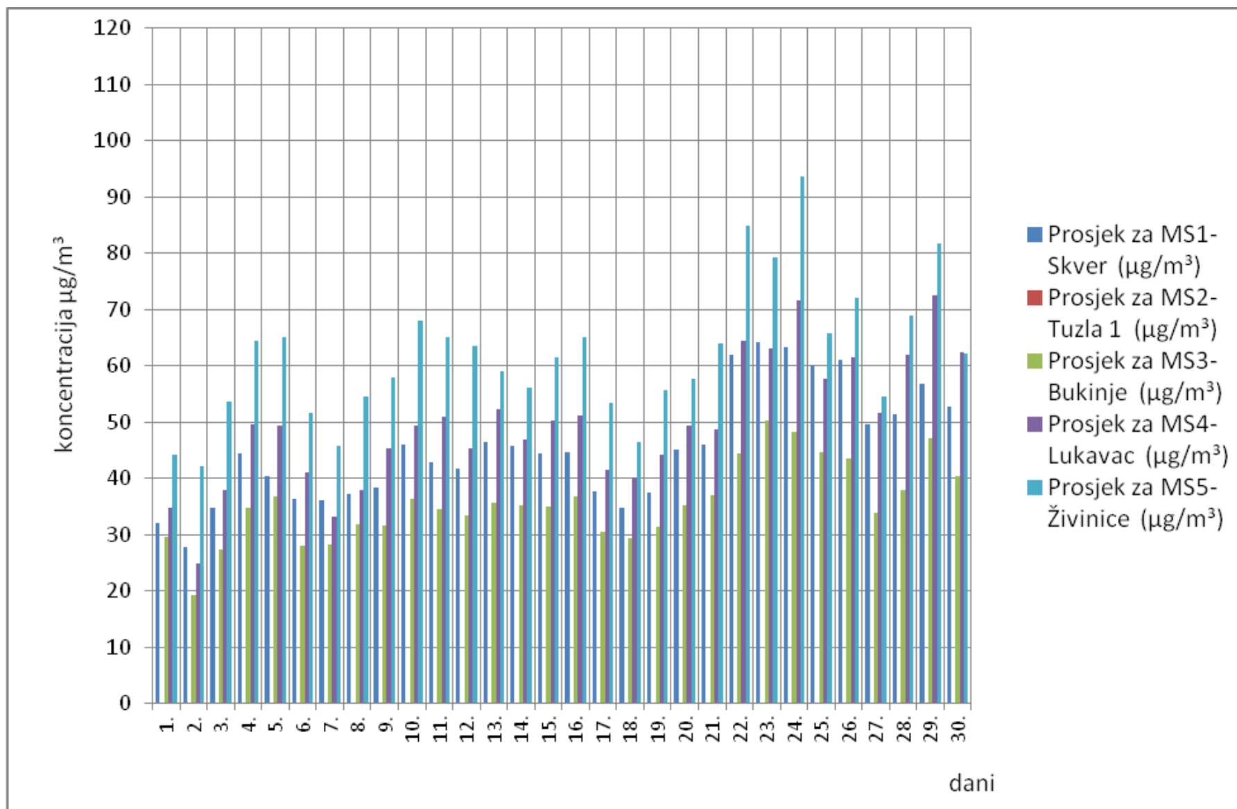
Slika 4. Grafički prikaz prosječnih dnevnih vrijednosti ozona ( \text{O}_3 ) za mjesec juni/lipanj 2017. godine
