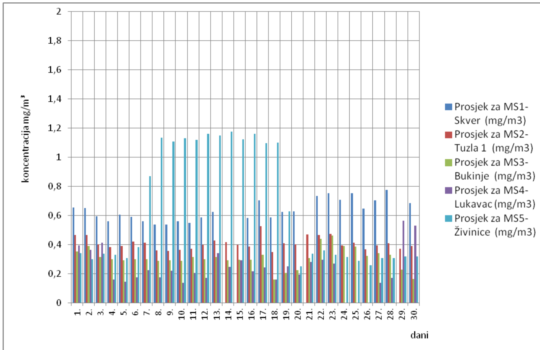
Slika 3. Grafički prikaz prosječnih dnevnih vrijednosti ugljenmonoksida (CO) za mjesec juni/lipanj 2017. godine
