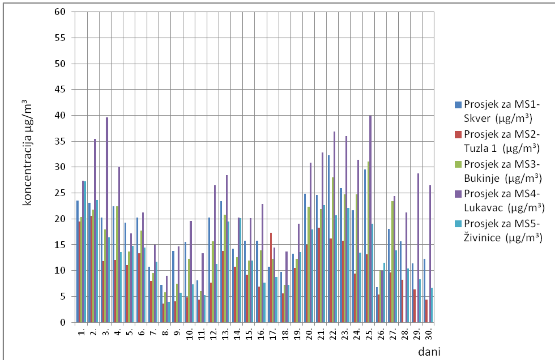
Slika 5. Grafički prikaz prosječnih dnevnih vrijednosti suspendovanih čestica ( \text{PM}_{2,5} ) za mjesec juni/lipanj 2017. godine
