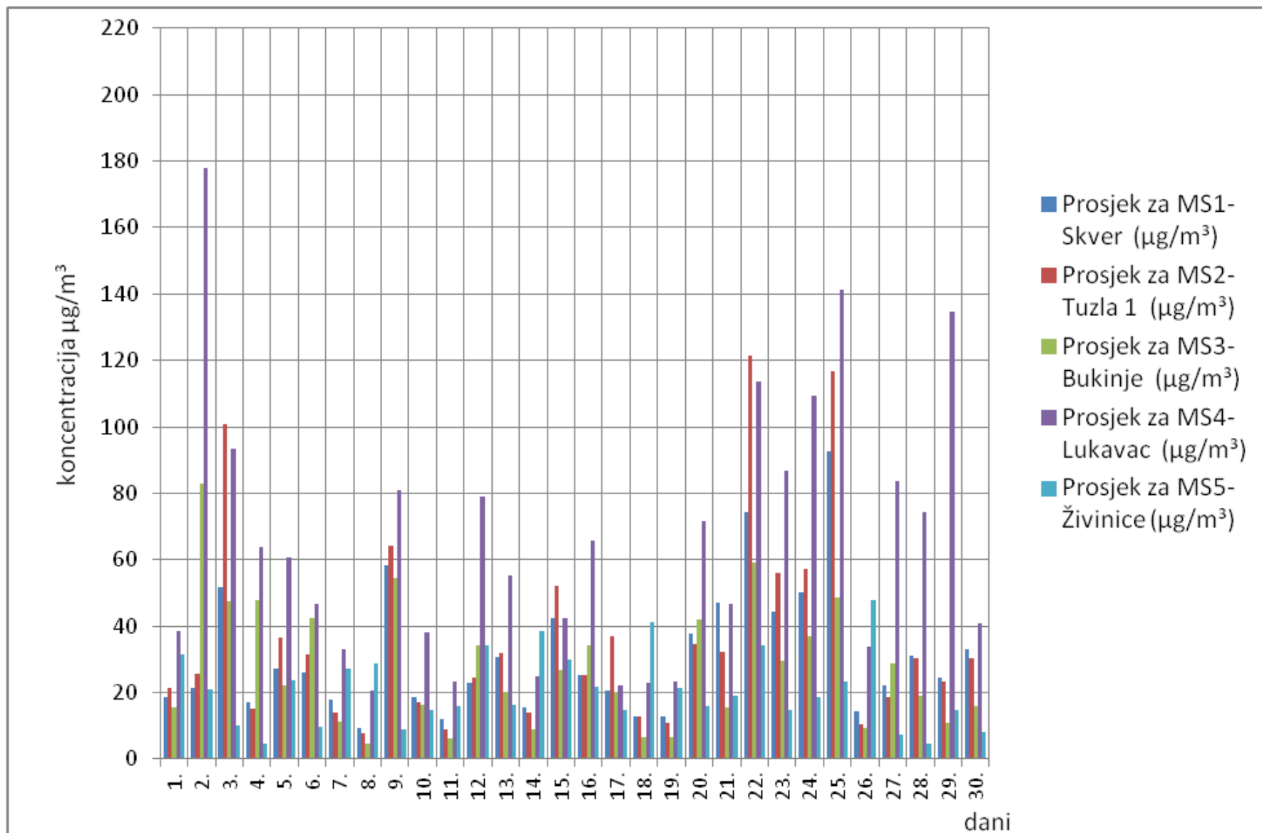
Slika 1. Grafički prikaz prosječnih dnevnih vrijednosti sumpordioksida (SO 2 ) za mjesec juni/lipanj 2017. godine
