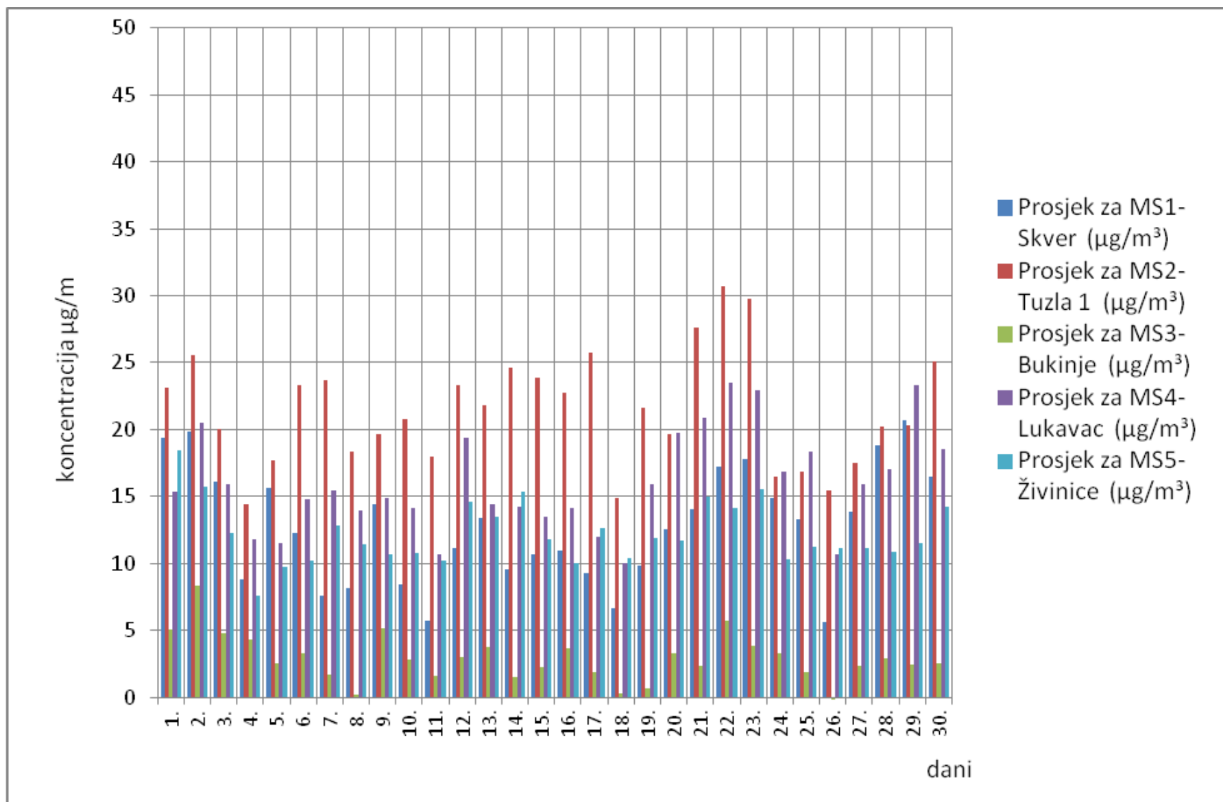
Slika 2. Grafički prikaz prosječnih dnevnih vrijednosti azotdioksida (NO 2 ) za mjesec juni/lipanj 2017. godine
