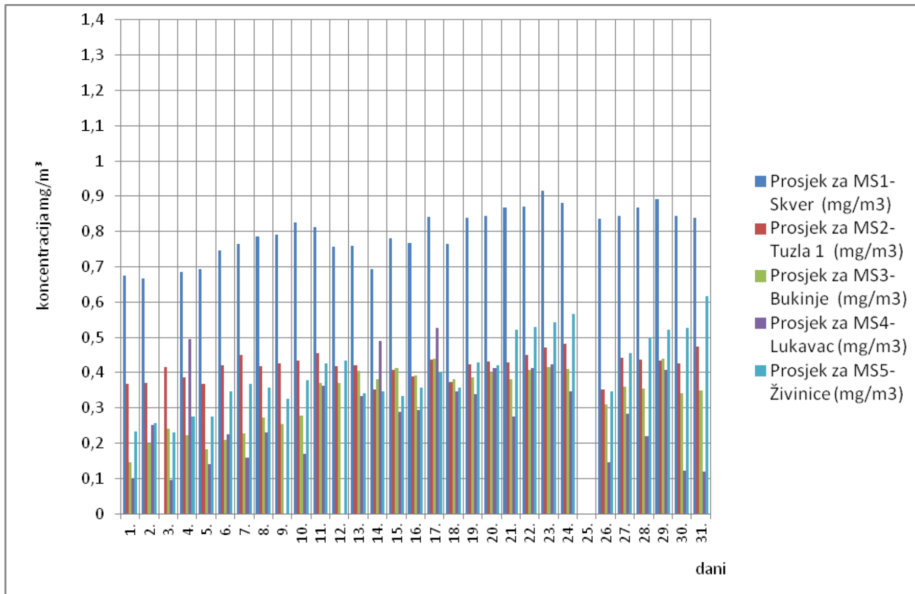
Slika 3. Grafički prikaz prosječnih dnevnih vrijednosti ugljenmonoksida (CO) za mjesec juli/srpanj 2017. godine
