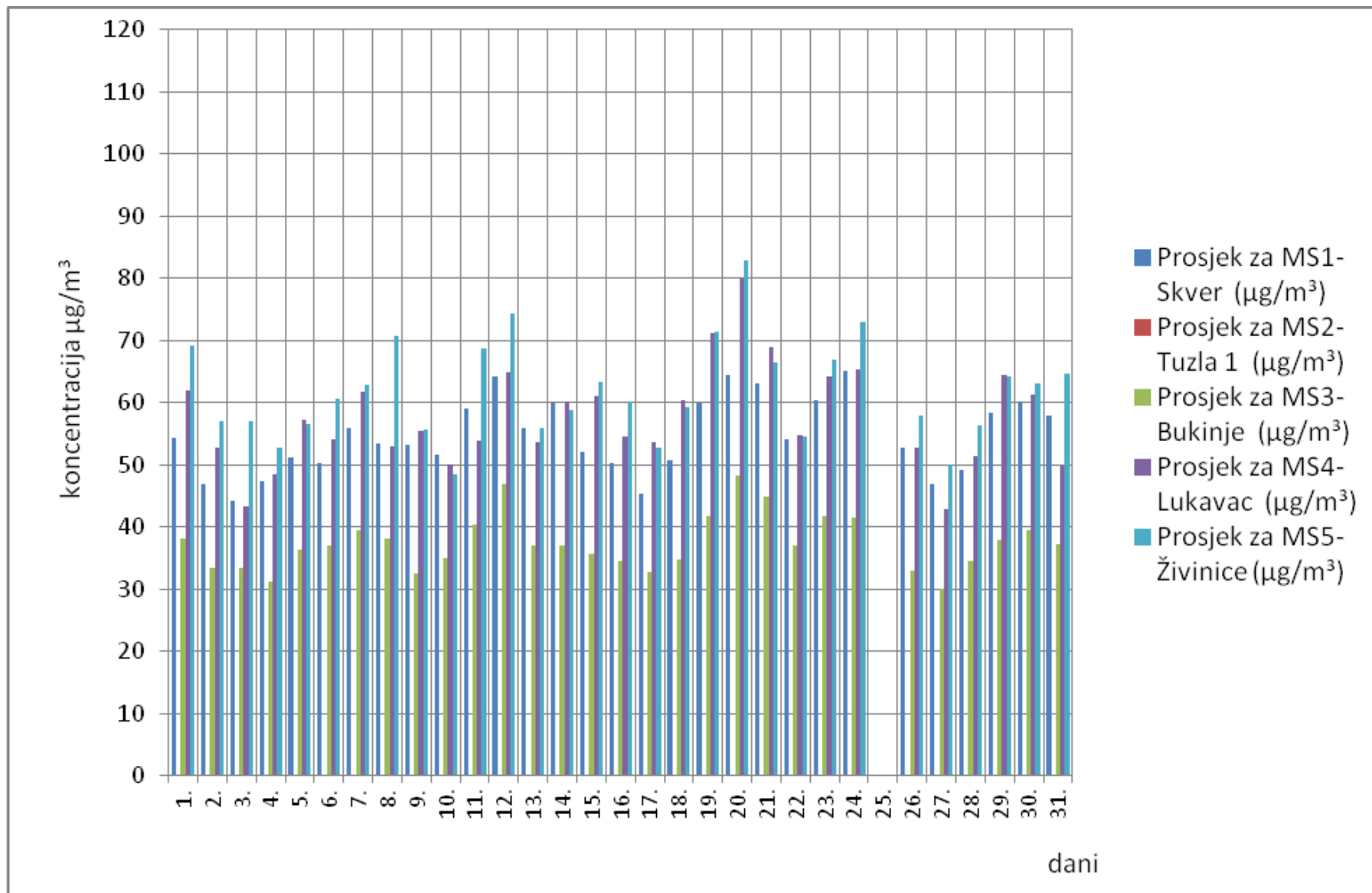
Slika 4. Grafički prikaz prosječnih dnevnih vrijednosti ozona ( \text{O}_3 ) za mjesec juli/srpanj 2017. godine
