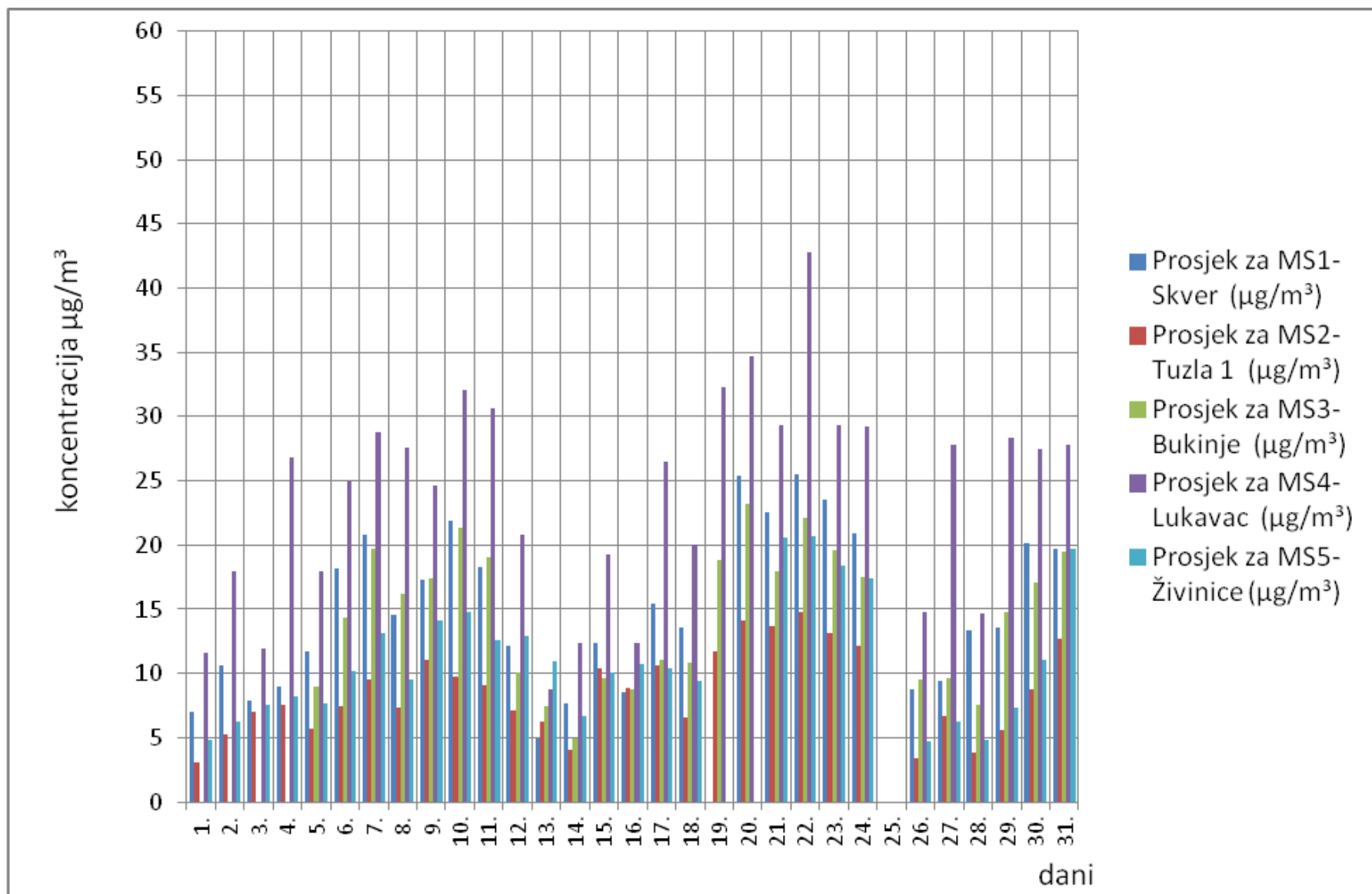
Slika 5. Grafički prikaz prosječnih dnevnih vrijednosti suspendovanih čestica (PM 2,5 ) za mjesec juli/srpanj 2017. godine
