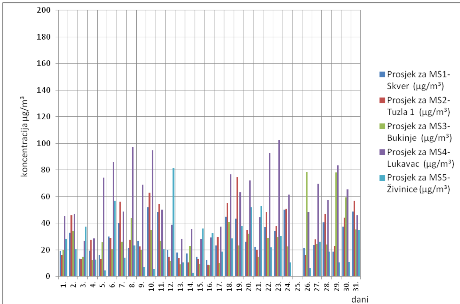
Slika 1. Grafički prikaz prosječnih dnevnih vrijednosti sumpordioksida (SO 2 ) za mjesec juli/srpanj 2017. godine
