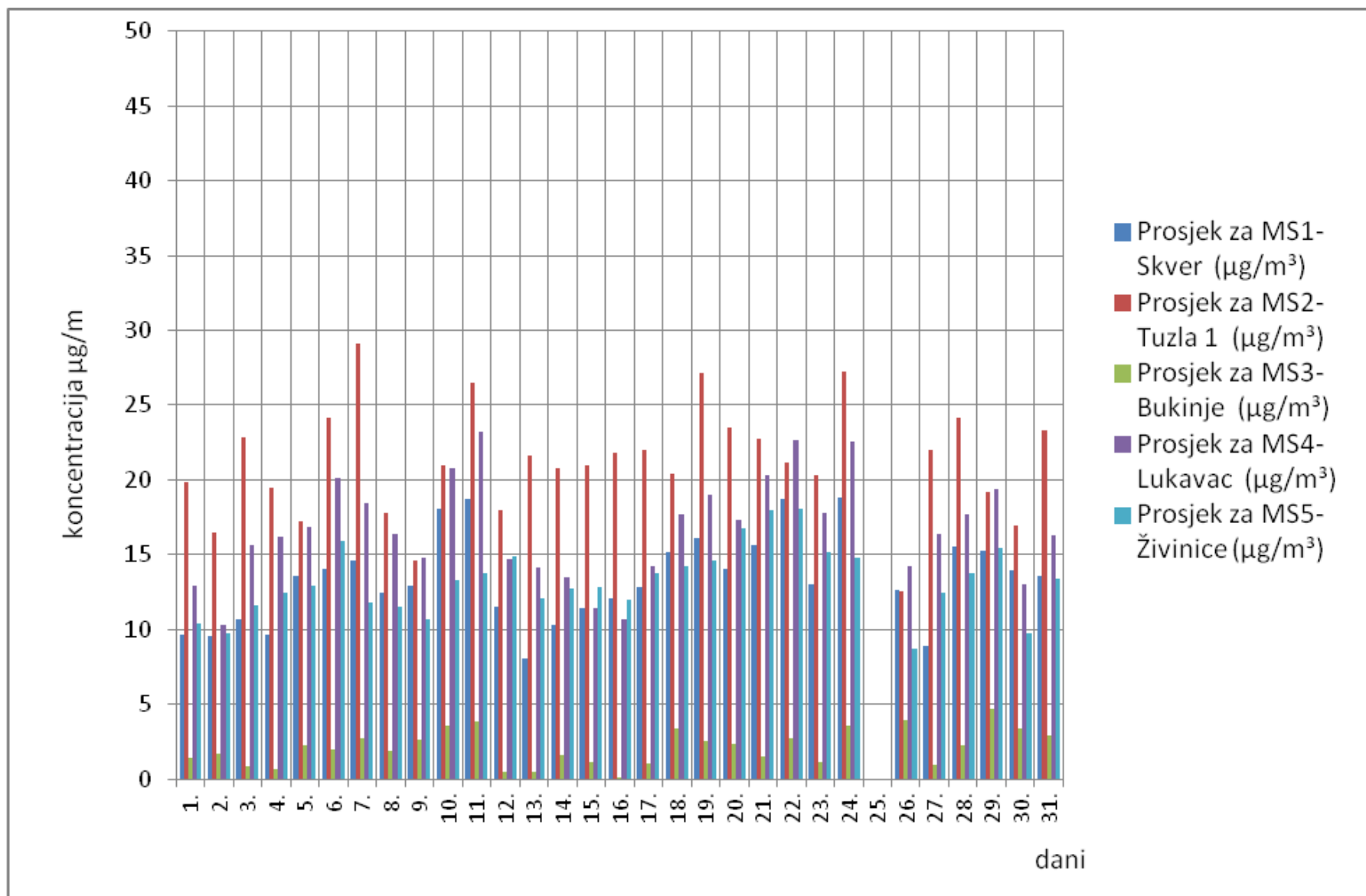
Slika 2. Grafički prikaz prosječnih dnevnih vrijednosti azotdioksida (NO 2 ) za mjesec juli/srpanj 2017. godine
