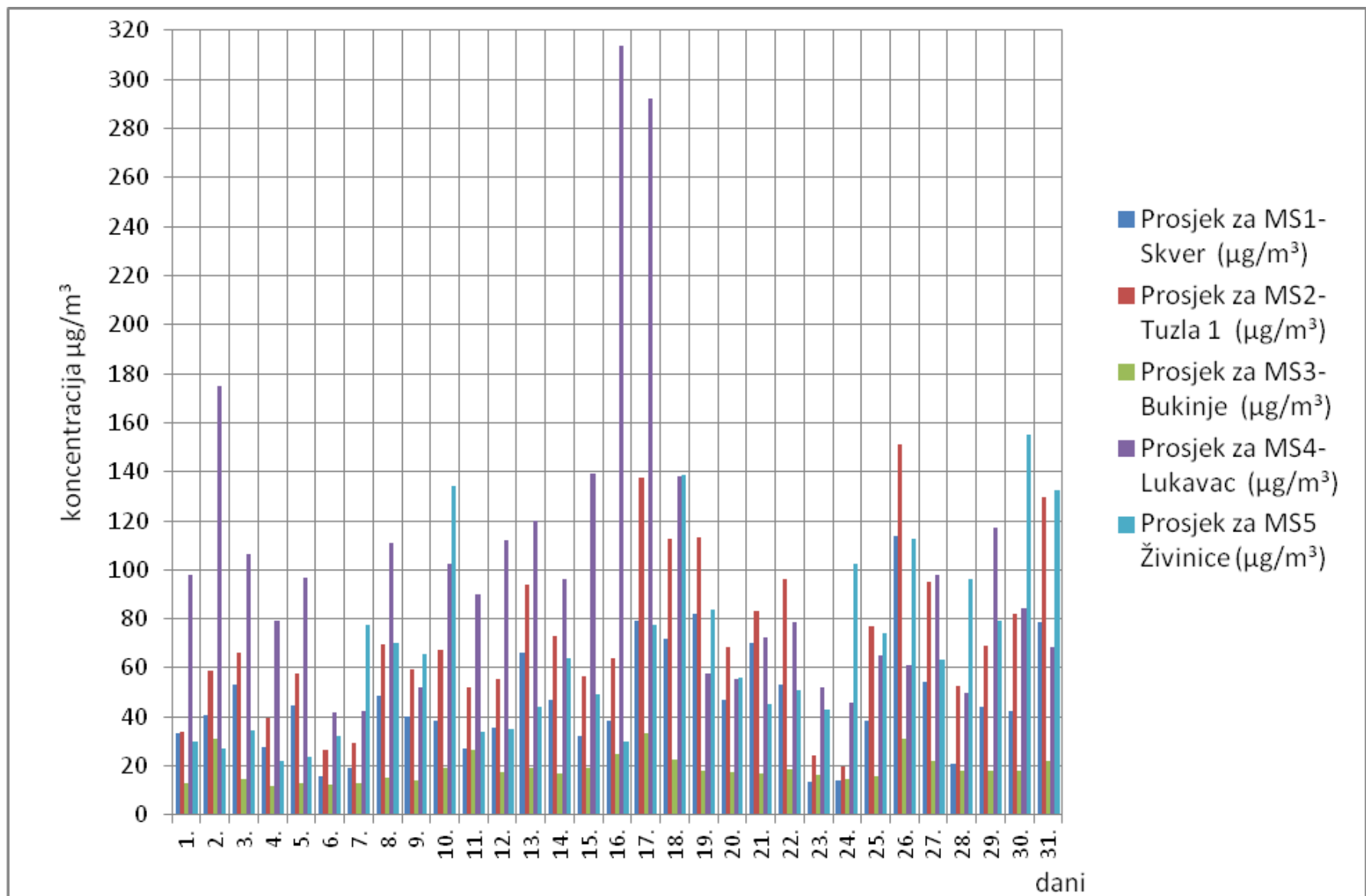
Slika 1. Grafički prikaz prosječnih dnevnih vrijednosti sumpordioksida (SO 2 ) za mjesec oktobar/listopad 2017. godine
