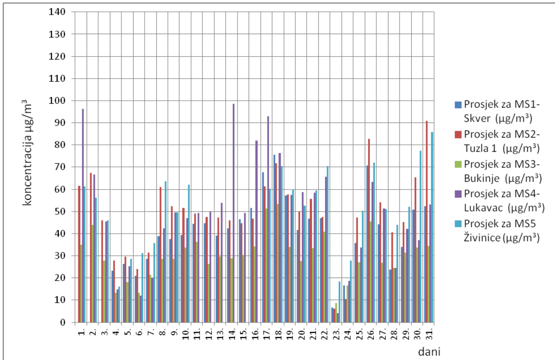
Slika 5. Grafički prikaz prosječnih dnevnih vrijednosti suspendovanih čestica (PM 2,5 ) za mjesec oktobar/listopad 2017. godine
