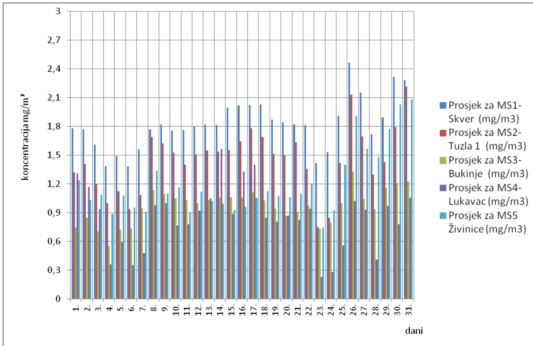
Slika 3. Grafički prikaz prosječnih dnevnih vrijednosti ugljenmonoksida (CO) za mjesec oktobar/listopad 2017. godine
