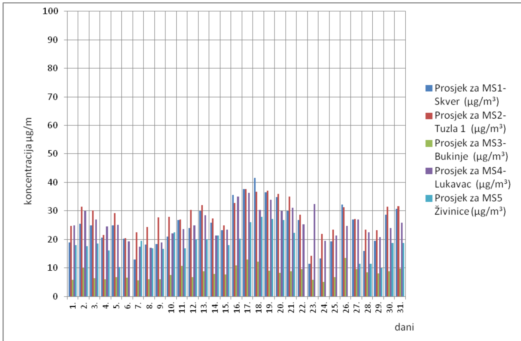
Slika 2. Grafički prikaz prosječnih dnevnih vrijednosti azotdioksida (NO 2 ) za mjesec oktobar/listopad 2017. godine
