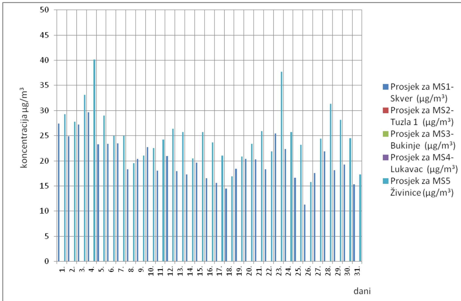
Slika 4. Grafički prikaz prosječnih dnevnih vrijednosti ozona ( \text{O}_3 ) za mjesec oktobar/listopad 2017. godine
