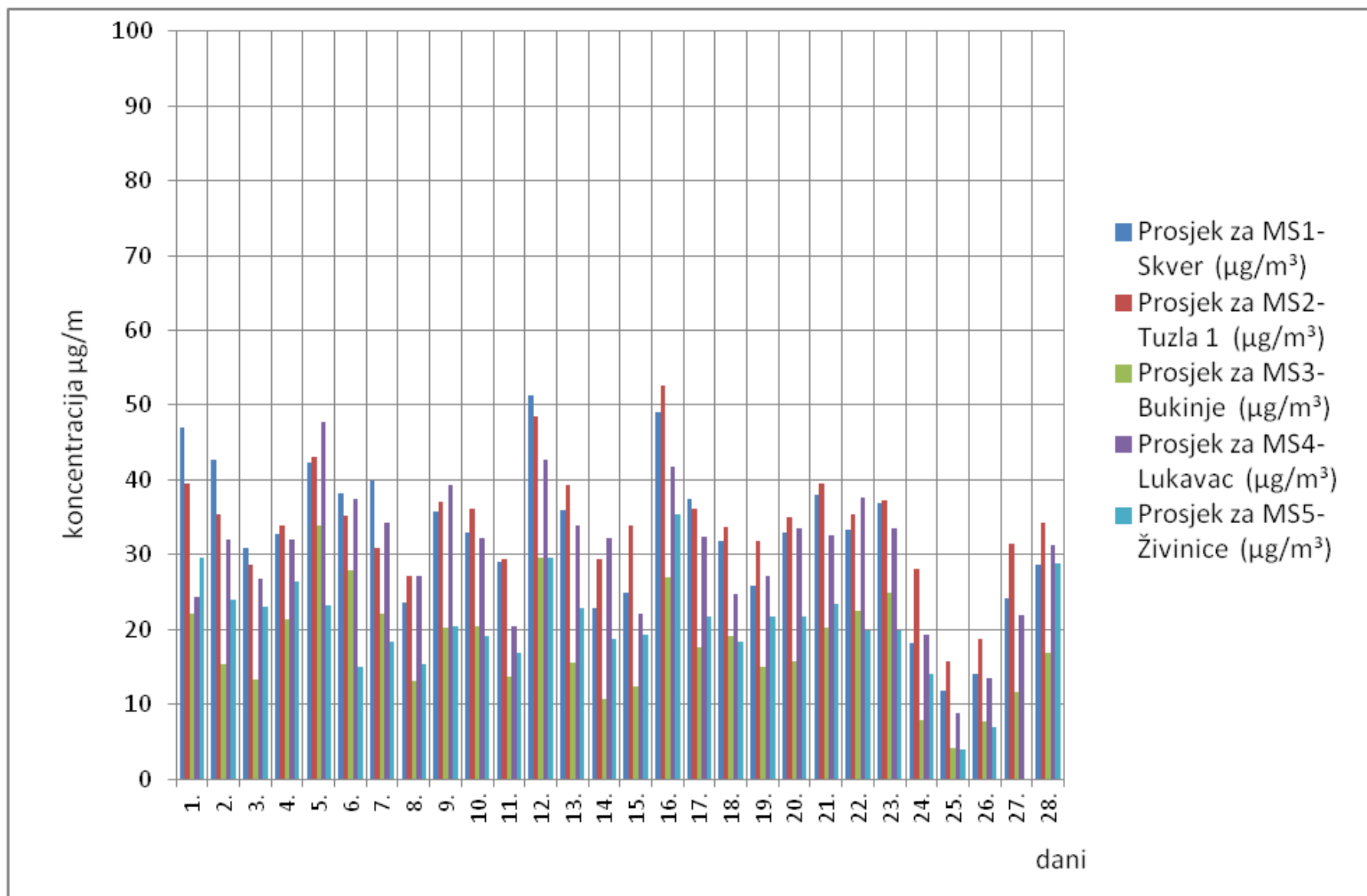
Slika 2. Grafički prikaz prosječnih dnevnih vrijednosti azotdioksida (NO 2 ) za mjesec februar/veljača 2018. godine
