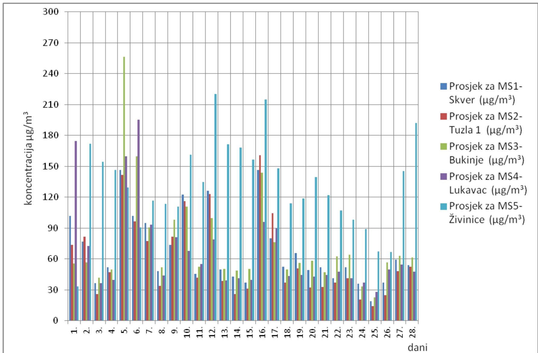
Slika 1. Grafički prikaz prosječnih dnevnih vrijednosti sumpordioksida (SO 2 ) za mjesec februar/veljača 2018. godine
