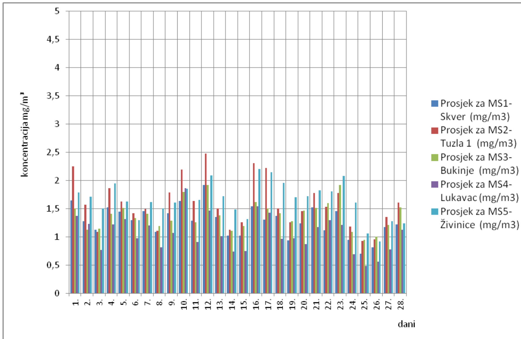
Slika 3. Grafički prikaz prosječnih dnevnih vrijednosti ugljenmonoksida (CO) za mjesec februar/veljača 2018. godine
