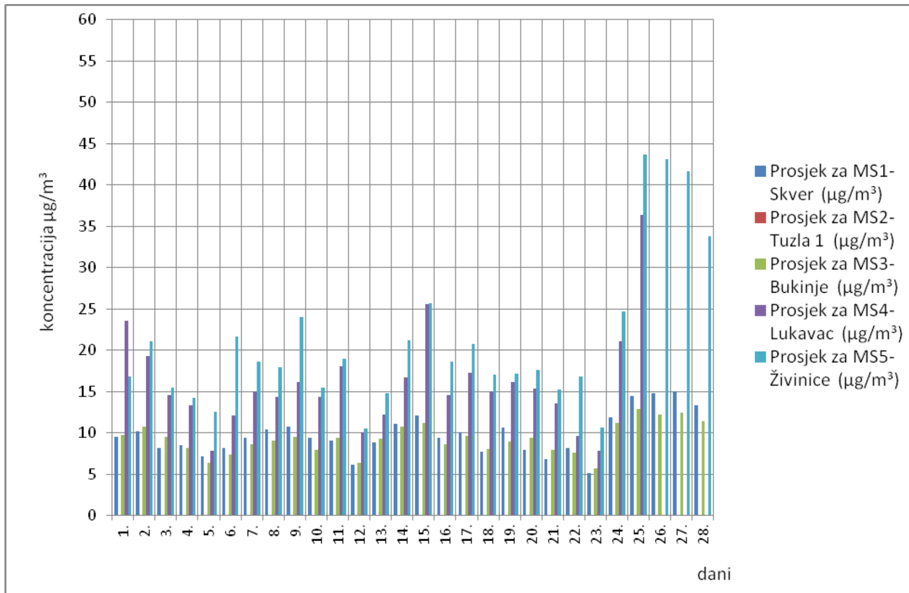
Slika 4. Grafički prikaz prosječnih dnevnih vrijednosti ozona (O 3 ) za mjesec februar/veljača 2018. godine
