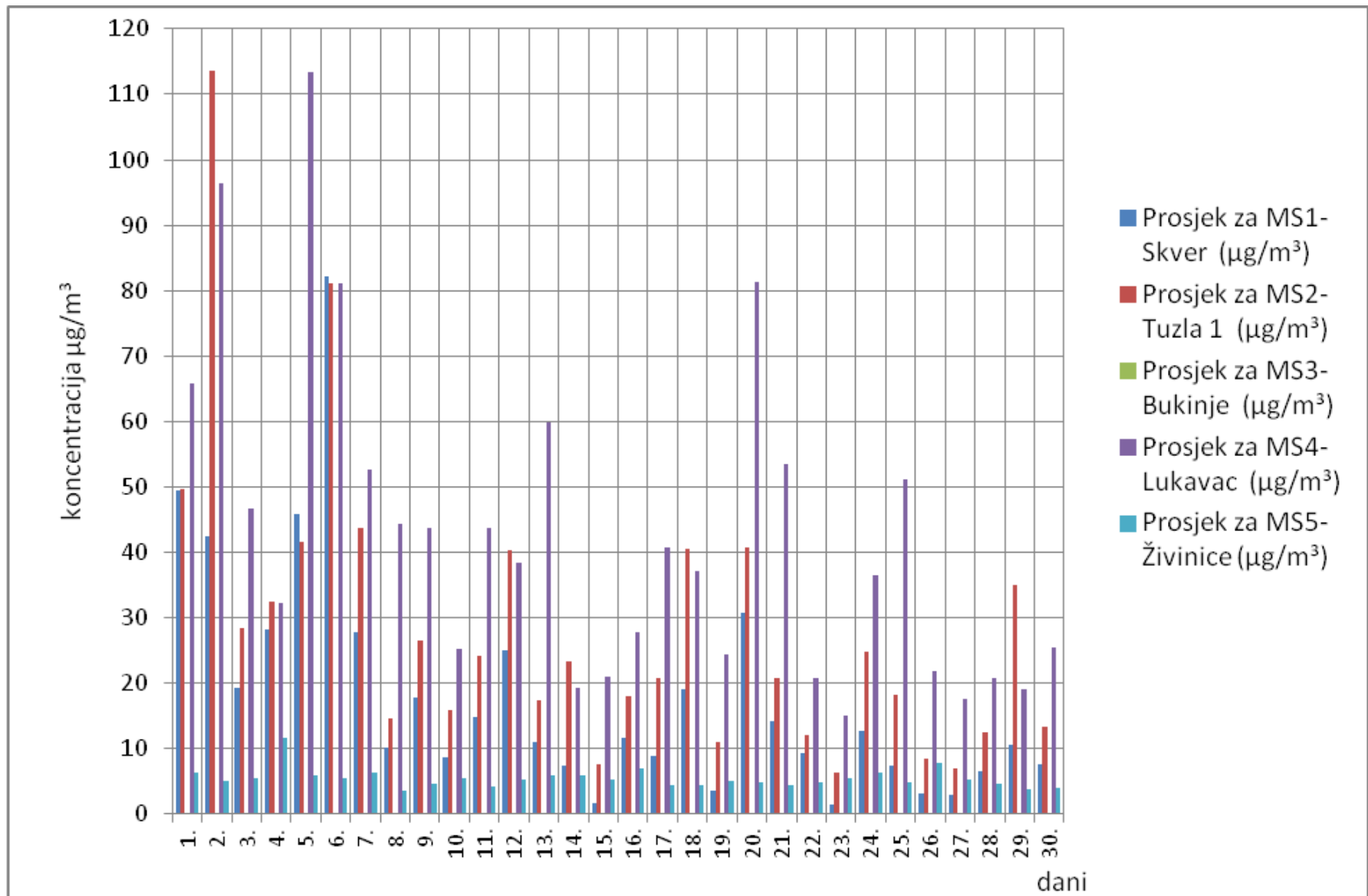
Slika 1. Grafički prikaz prosječnih dnevnih vrijednosti sumpordioksida (SO 2 ) za mjesec juni/lipanj 2018. godine
