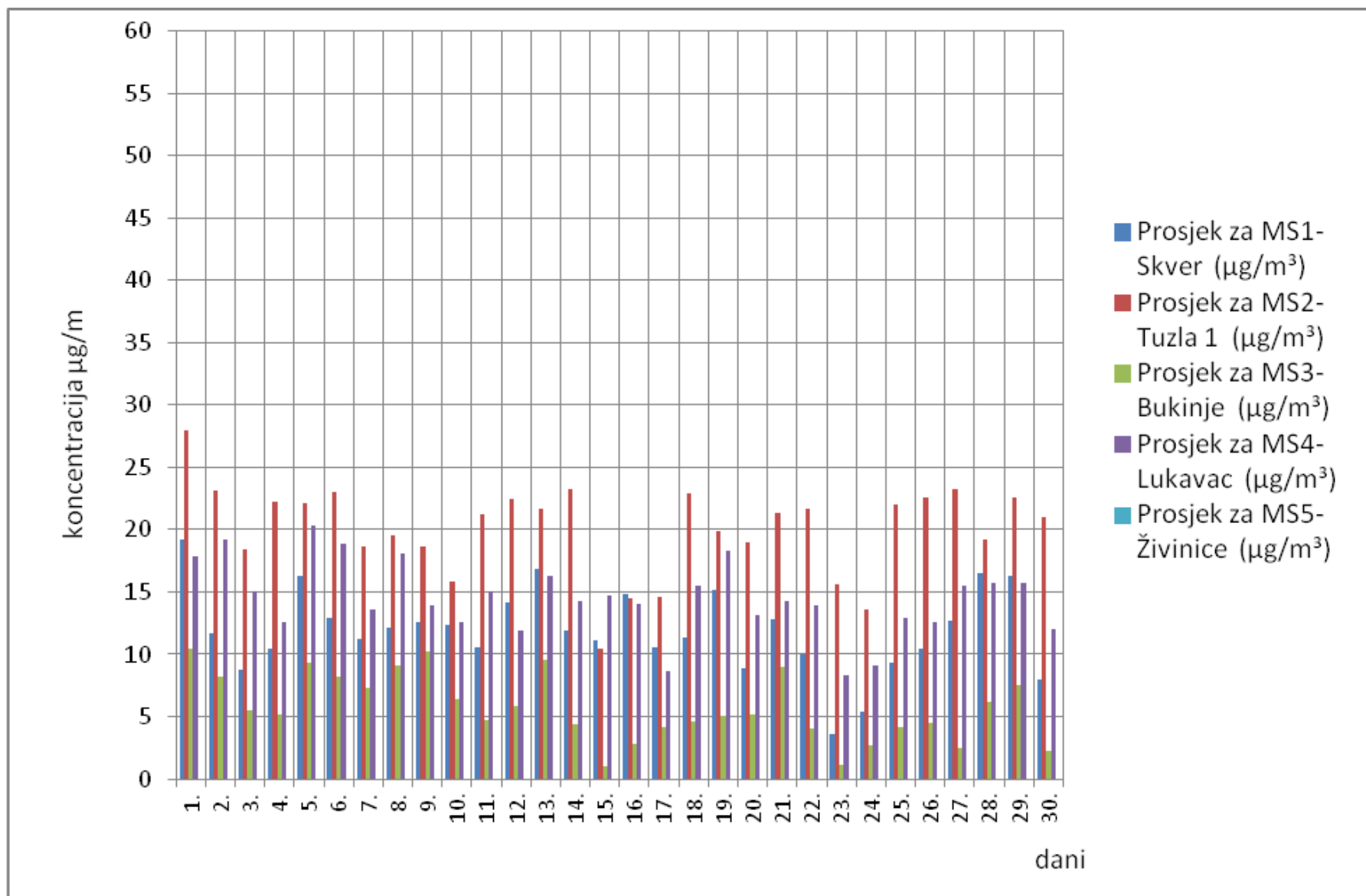
Slika 2. Grafički prikaz prosječnih dnevnih vrijednosti azotdioksida (NO 2 ) za mjesec juni/lipanj 2018. godine
