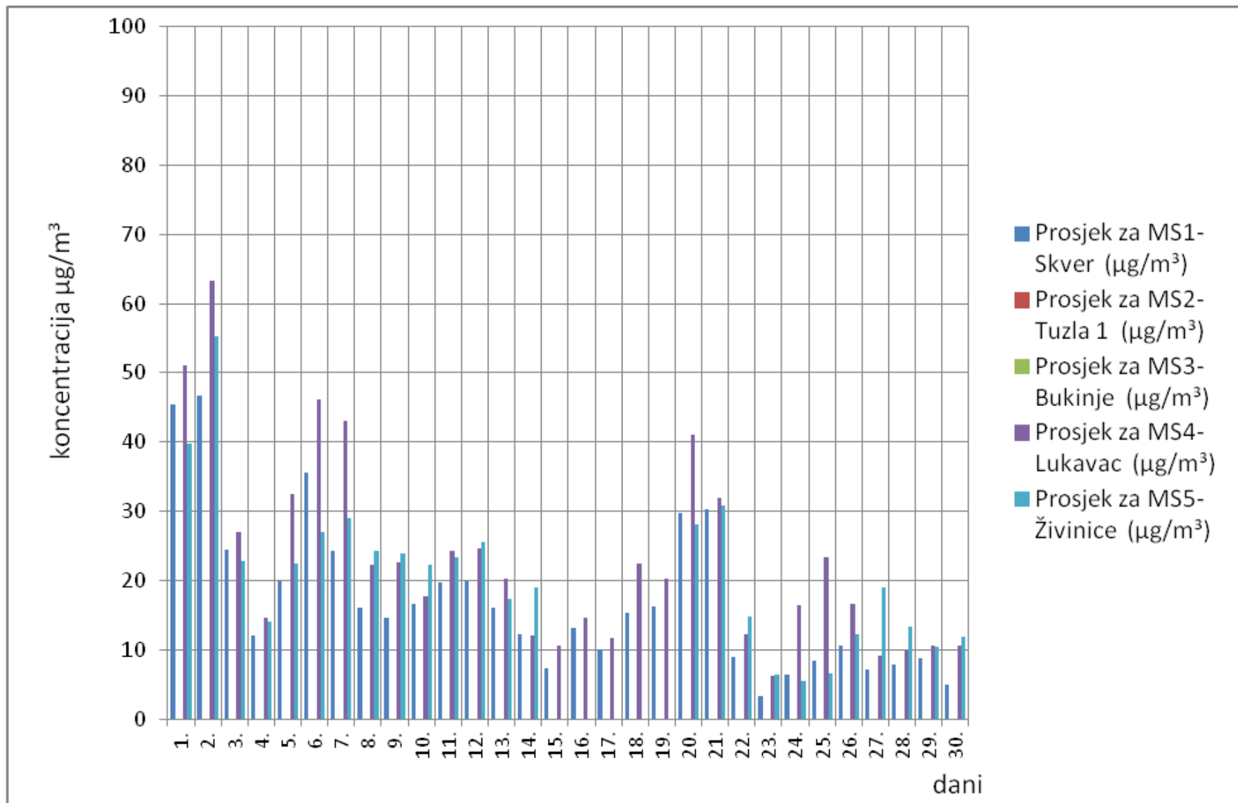
Slika 5. Grafički prikaz prosječnih dnevnih vrijednosti suspendovanih čestica (PM 2,5 ) za mjesec juni/lipanj 2018. godine
