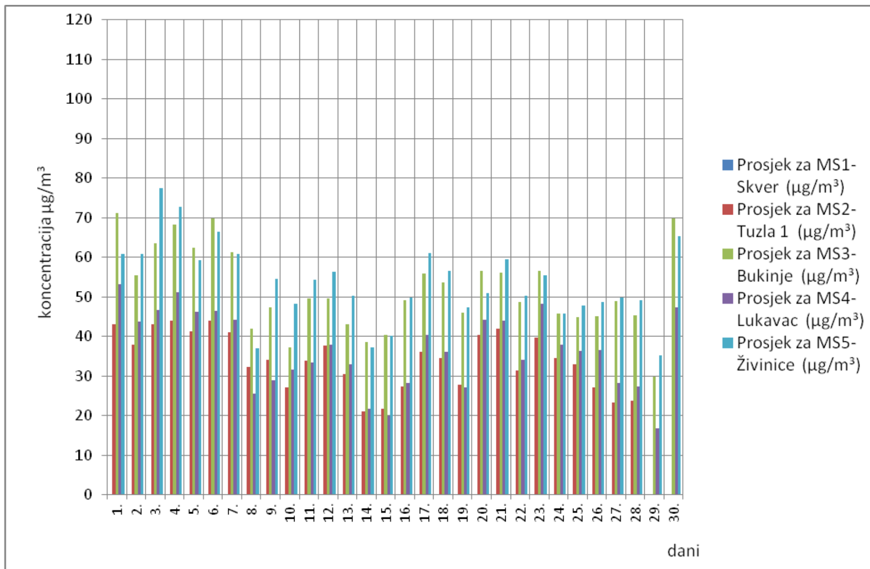
Slika 4. Grafički prikaz prosječnih dnevnih vrijednosti ozona ( \text{O}_3 ) za mjesec juni/lipanj 2018. godine
