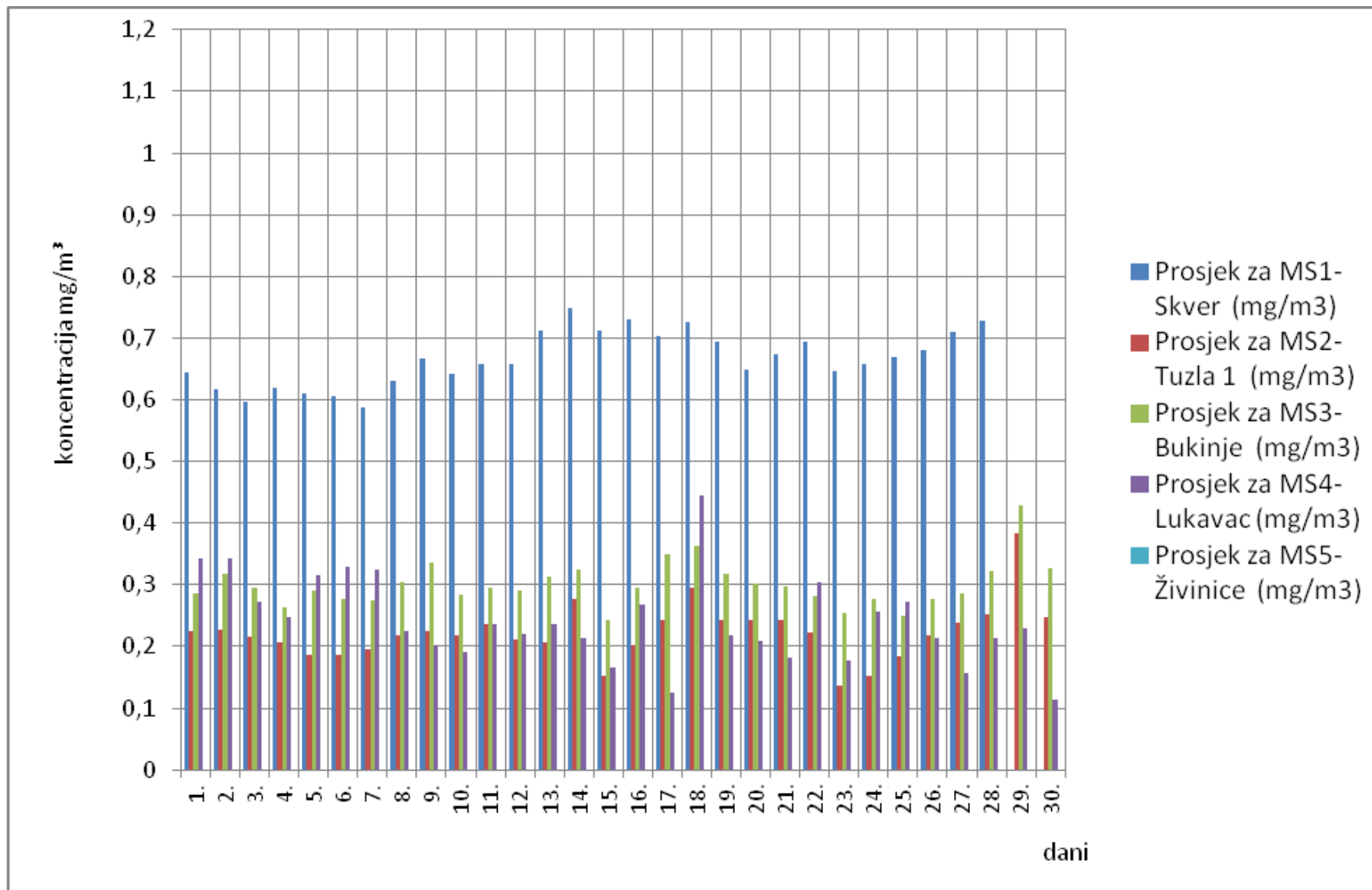
Slika 3. Grafički prikaz prosječnih dnevnih vrijednosti ugljenmonoksida (CO) za mjesec juni/lipanj 2018. godine
